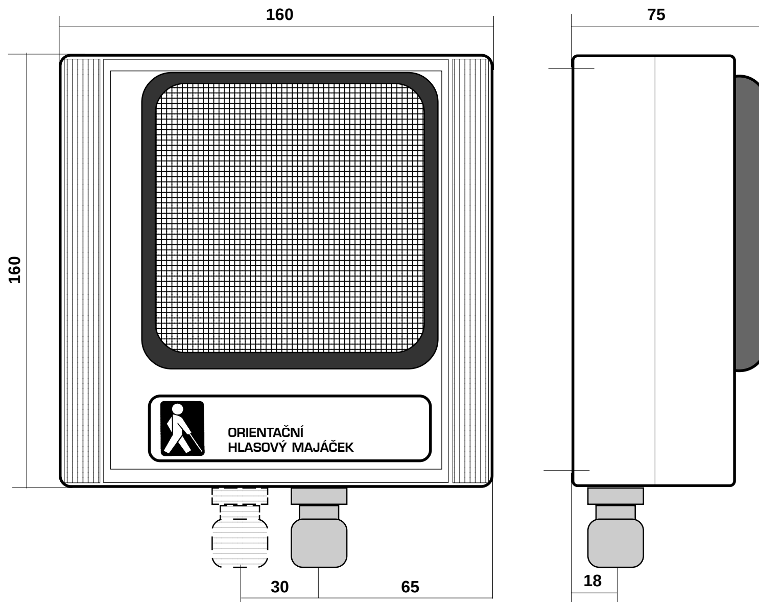
ORIENTAČNÍ HLASOVÝ MAJÁČEK ELVOS OHM (ZE ZADNÍ STRANY 4 MONTÁŽNÍ DÍRY V ROZTEČI 145X145mm)
